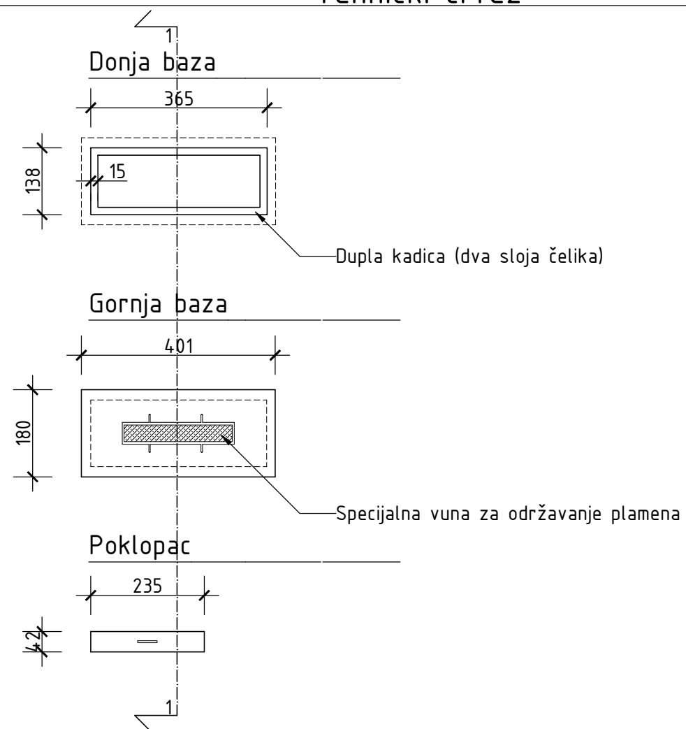
Presek kroz gorionik 1-1
