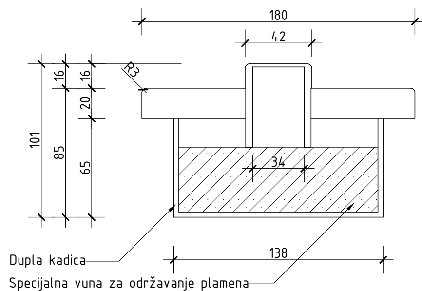
Presek kroz gorionik 1-1
